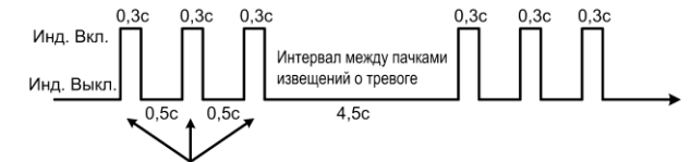
Рис.1 Работа индикатора в режиме «Память тревог»
