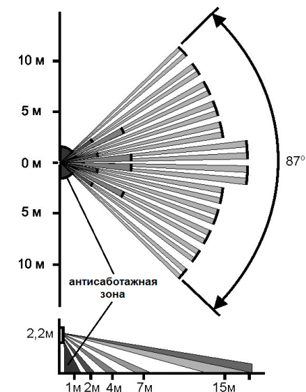
Рис.4 Диаграмма зоны обнаружения при установке извещателя на высоту 2,2 м и наклоне основания извещателя вниз (в вертикальной плоскости) на угол 12°
