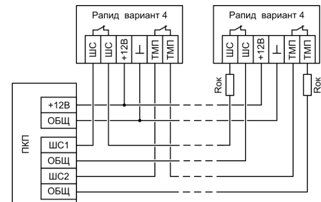
Рис.3 Схема подключения извещателей к ПКП
